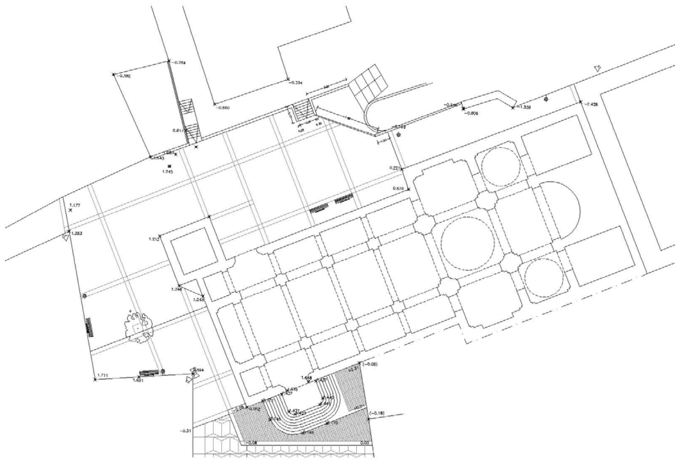
Planta
