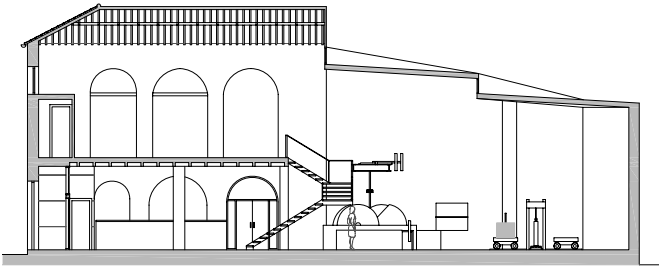
Sección longitudinal
