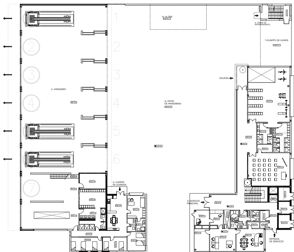
Planta baja
