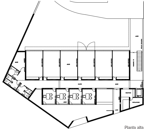
Planta alta
