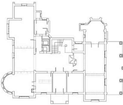
Planta baja
