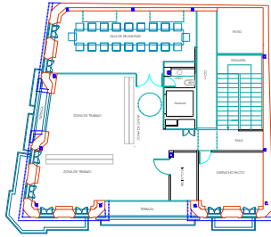
PLANTA SEGUNDA
