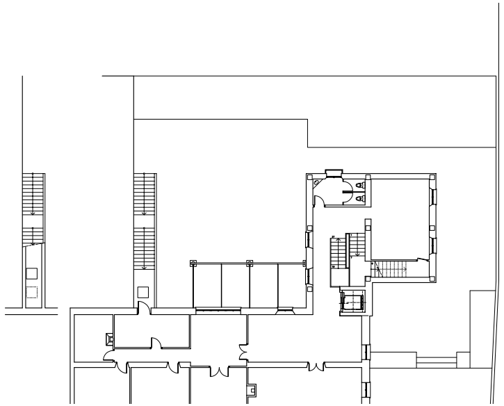
Planta baja
