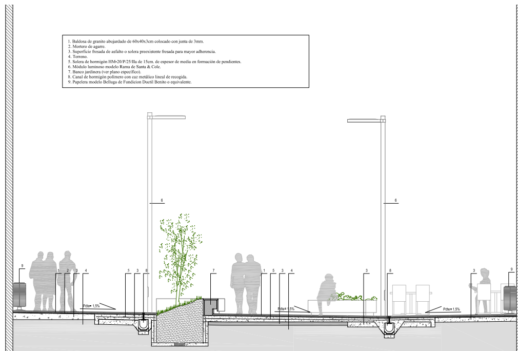
Sección transversal
