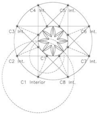
Trazado Estrella de la Catedral
