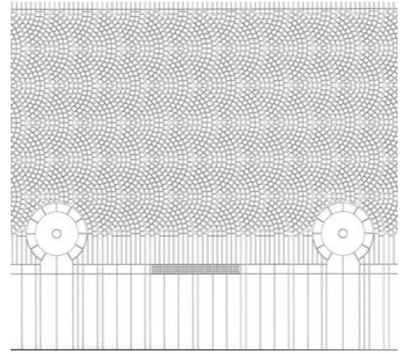
Detalles Calles Strachan y Bolsa
